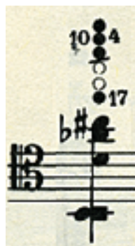
Fagott Takt 11
