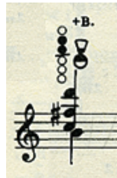
Oboe 1 Takt 51
